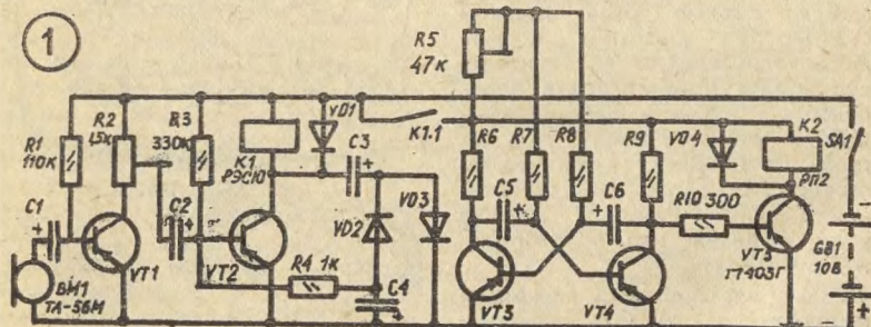
Рисунок 1. Принципиальная схема электронной погремушки.
